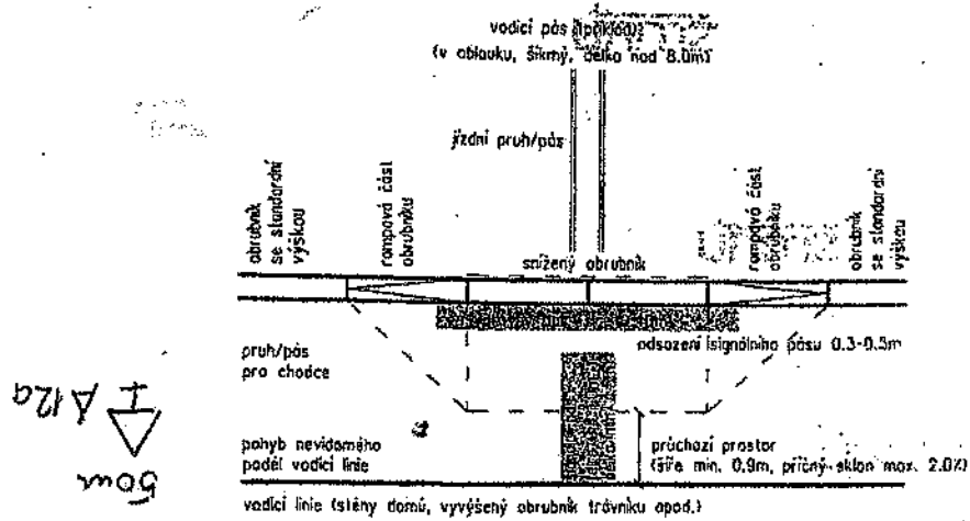
Obrázek 50 – Místo pro přecházení – standardní hmatové úpravy
